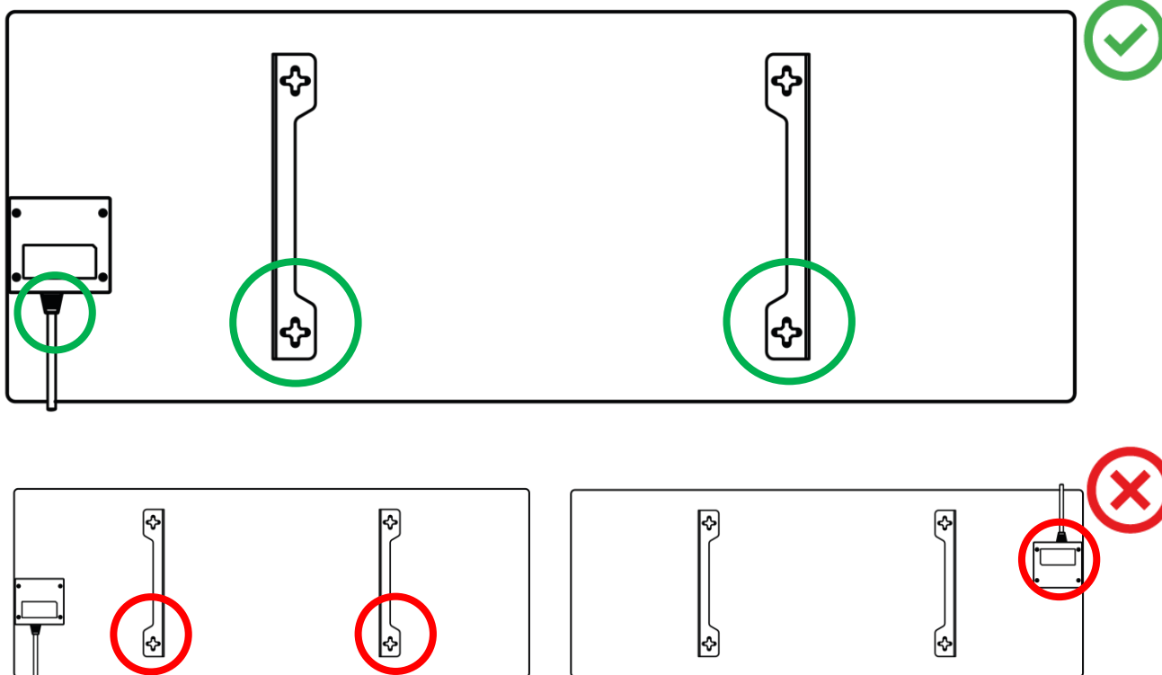
Obrázek 7 – Instalace držáků
