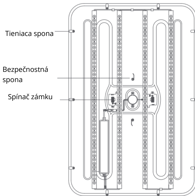
Základná doska
