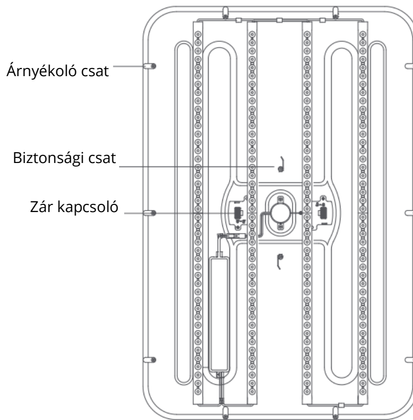
Alaplemez
