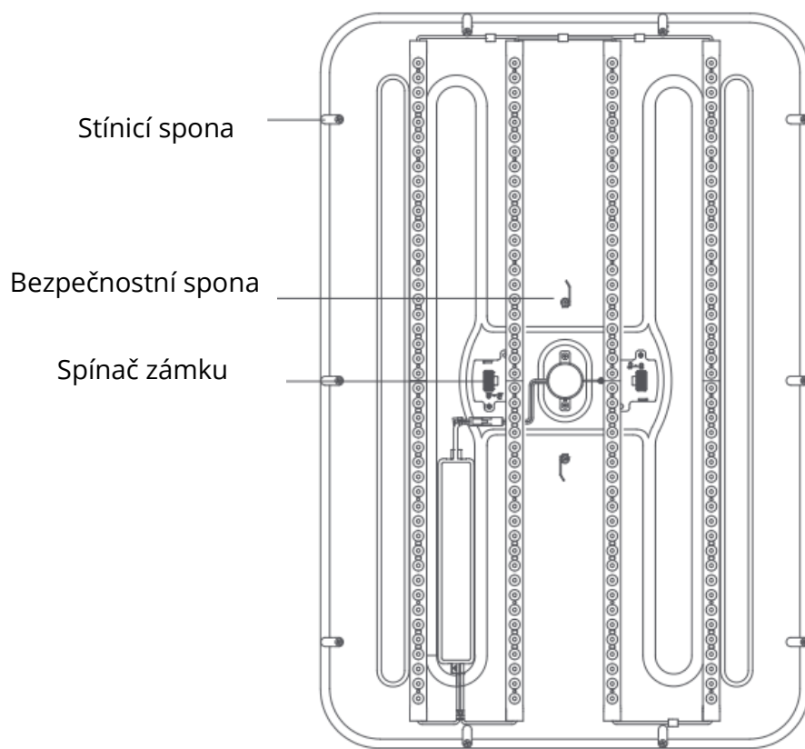
Základní deska
