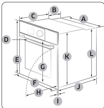
Trouba (mm)
