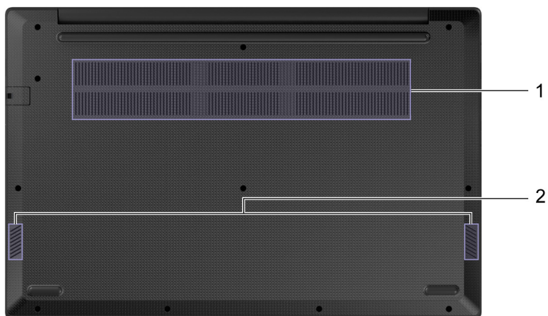
Obrázek 9. Pohled zespodu – 15" modely
