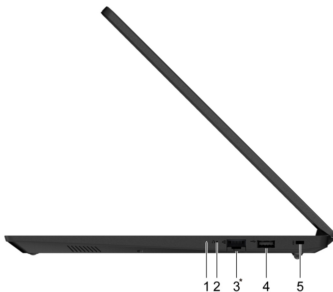
Obrázek 7. Pohled z pravé strany—15" modely
