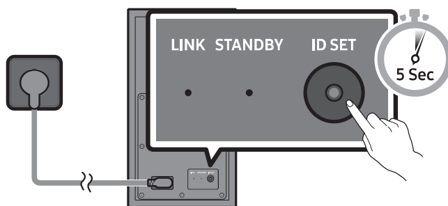
Zadná strana subwoofera
